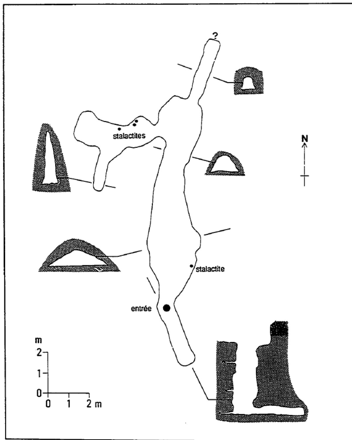
Figure 7.5: Topographie, Gouffre des Vents.
