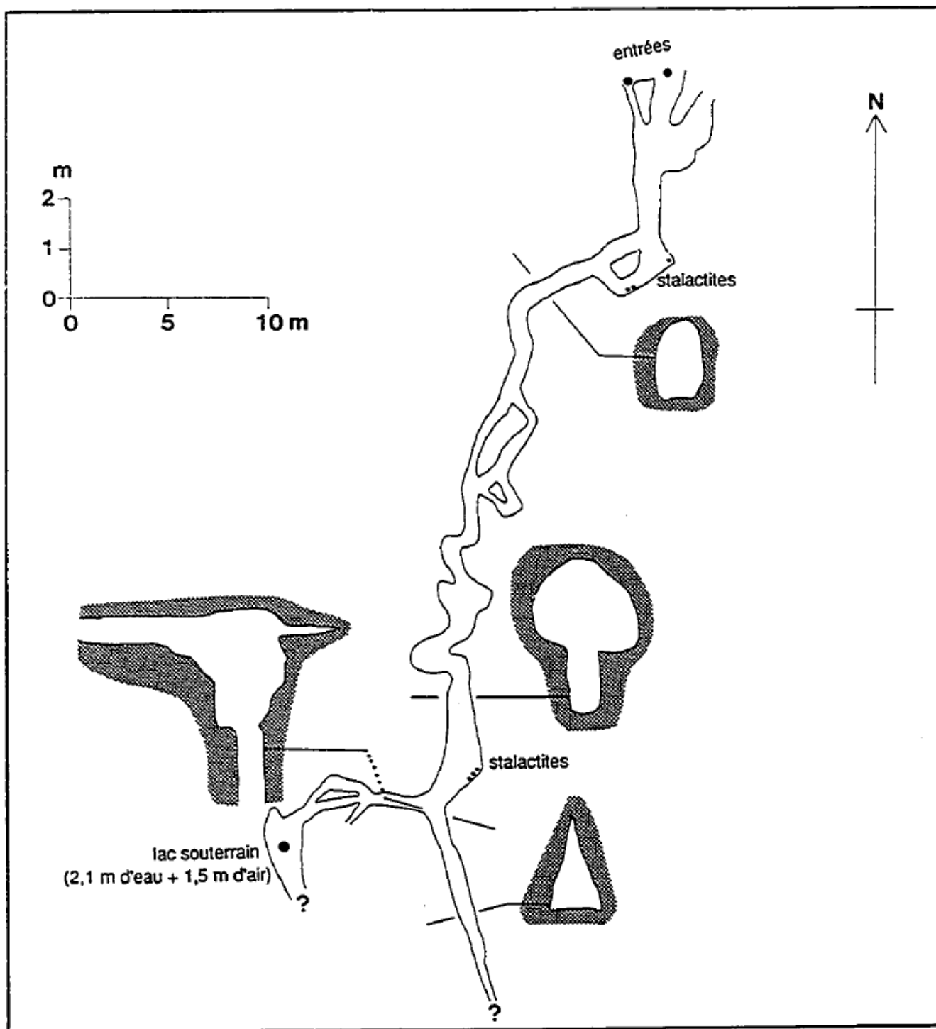
Figure 7.4: Topographie, Grotte du Marais (lac Samlock).
