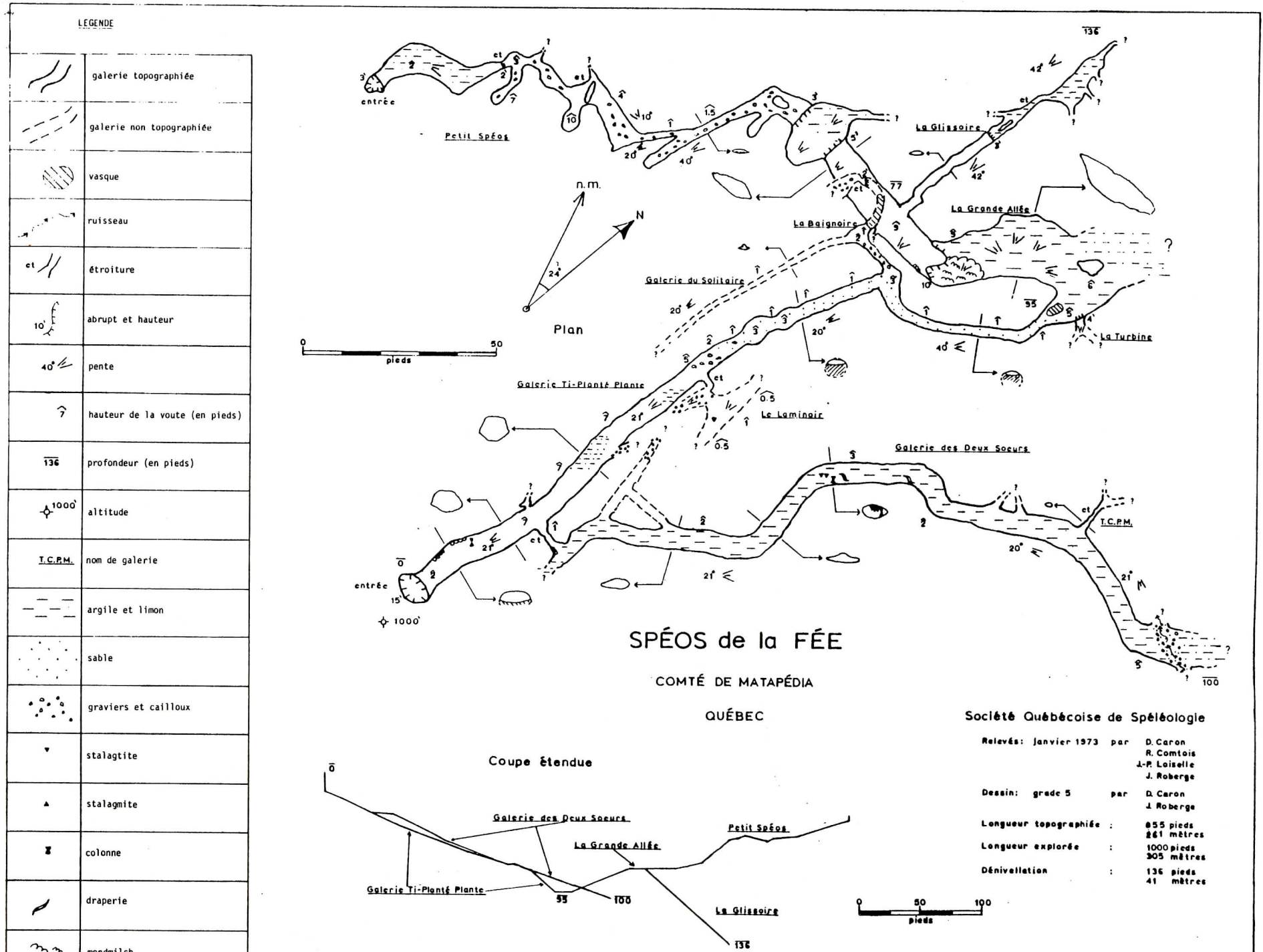
Figure 11 - Le plan du Spéos de la Fée.
